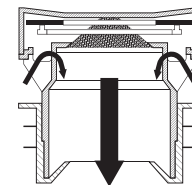
Открытый клапан
